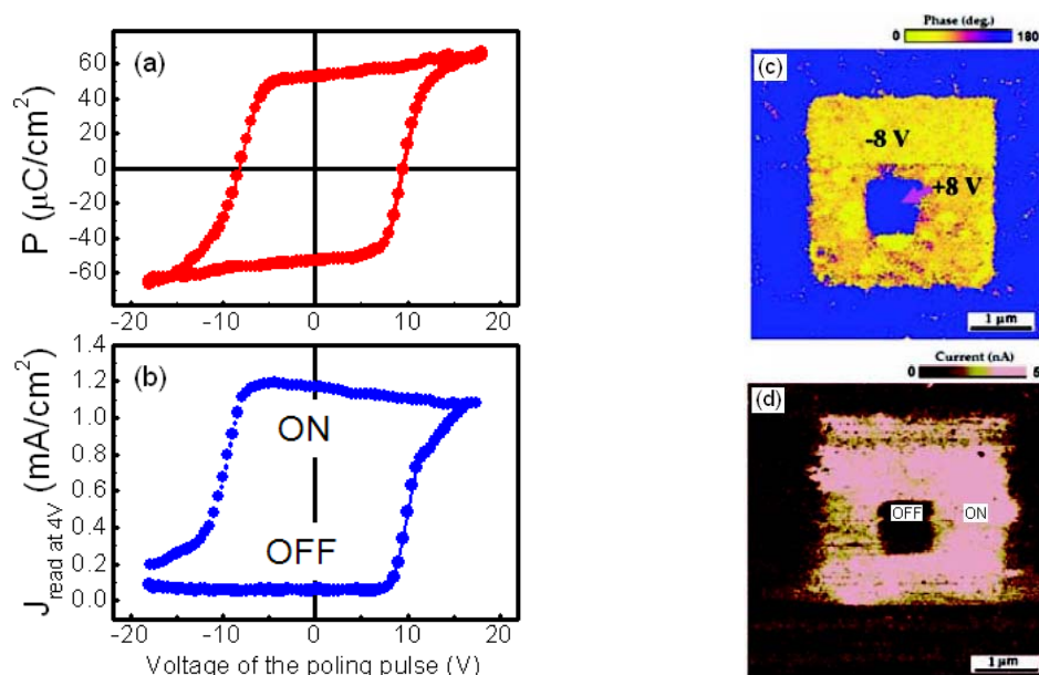
图 3. BFO 外延薄膜的电阻依赖铁电极化变化的证据。(a) 不同脉冲电压下测量的剩余极化强度(脉冲电压幅度从-20V 到 20V, 再到-20V); (b) 施加不同幅度脉冲电压后, 在 4V 测量的电流密度, 表示 BFO 的电阻改变对应着铁电极化强度的变化。(c)BFO 外延薄膜的压电力显微图(PFM), 实现局部微区的不同极化状态;(d)导电原子力显微图片(Conductive AFM),表示 BFO 薄膜微区的电阻随极化状态的不同而改变。
