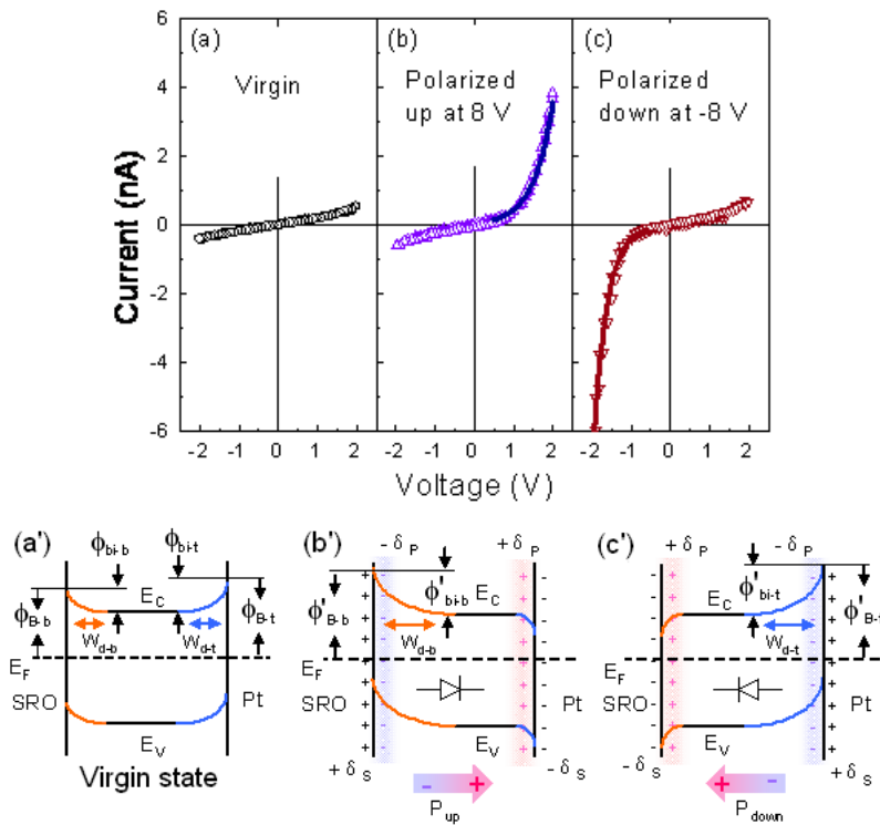
图 2. 可反转二极管特性与机制分析。(a)(b)(c)分别表示 BFO 外延薄膜初始态、向上极化、向下极化三个状态的导电特性。外加脉冲电压极化后，薄膜的 IV 特性呈现二极管整流效应，二极管导电极性方向可随脉冲电压极性即铁电极化方向变化而发生改变。(a')(b')(c') 分别对应 BFO 薄膜不同极化状态下的能带示意图，表示受铁电极化调制的 Schottky 势是导致可反转二极管特性的主要机制。
