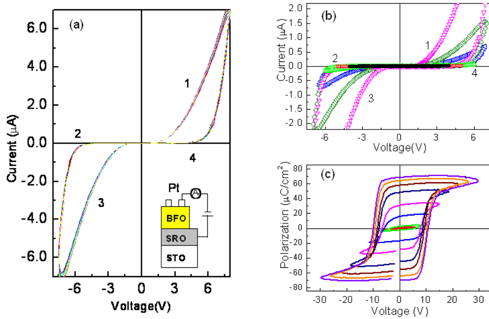
图 1. 电流电压(IV)关系曲线与铁电电滞回线。(a) BFO 外延薄膜的 IV 曲线，显著的回线特征表示 BFO 薄膜具有电致电阻特性，图中数字表示 IV 测量顺序。(b) IV 回线随测量电压增加逐渐增大。(c) BFO 外延薄膜的铁电极化回线。
